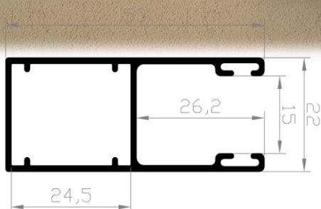
Standardlaufschiene A 3
