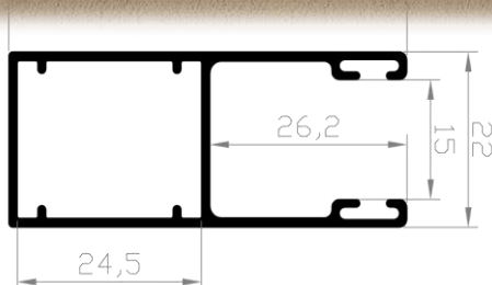
Standardlaufschiene A 3
