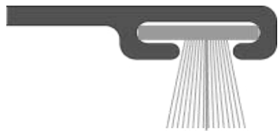
Laufschienen standartmässig mit Stabilbürsteneinlage ausgestattet
