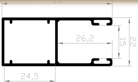
Standardlaufschiene A 3
