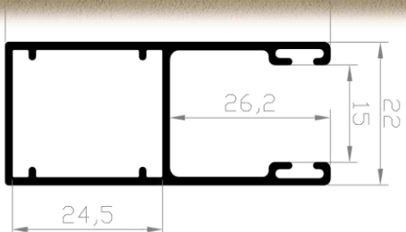
Standardlaufschiene A 3
