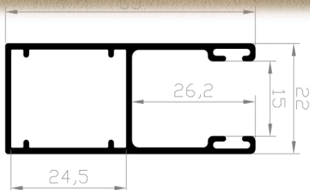
Standardlaufschiene A 3
