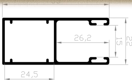
Standardlaufschiene A 3
